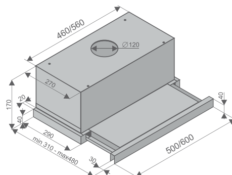
HELENA II / HELENA II GLASS ВСТРАИВАЕМЫЕ ТЕЛЕСКОПИЧЕСКИЕ
