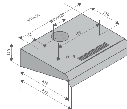
VERENA VERENA II КОЗЫРЬКОВЫЕ ПЛОСКИЕ
