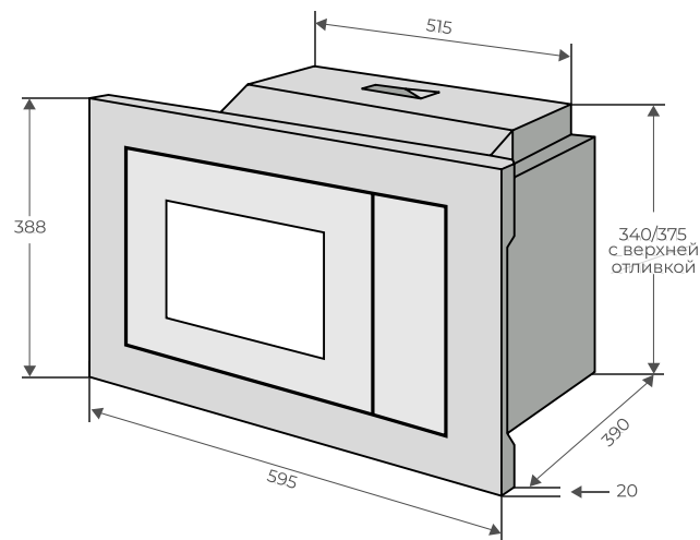
GTMB925BFG / GTMB925WG CB4
