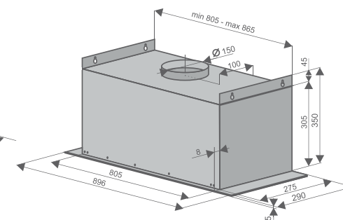
NAVI 90 ПОЛНОСТЬЮ ВСТРАИВАЕМЫЕ
