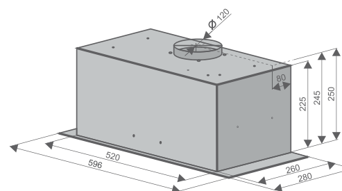
SKYBOX ПОЛНОСТЬЮ ВСТРАИВАЕМЫЕ
