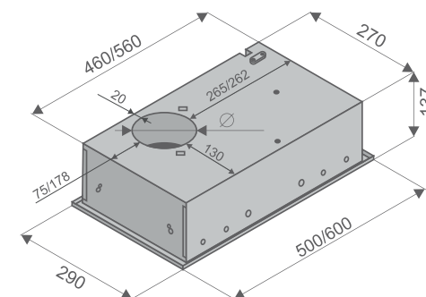
INBOX ПОЛНОСТЬЮ ВСТРАИВАЕМЫЕ
