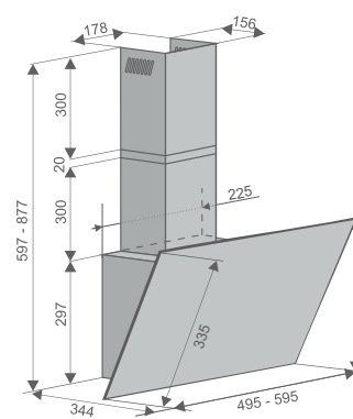
COLIBRI COLIBRI TECH НАСТЕННАЯ
