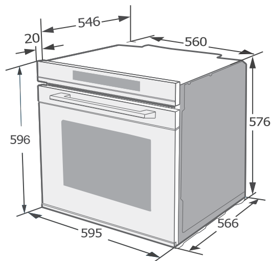
NEOS E13 ДУХОВЫЕ ШКАФЫ
