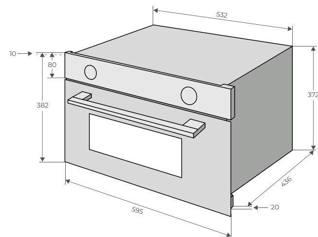
NEOS 60 BKF E934 / WH E934 CB4
