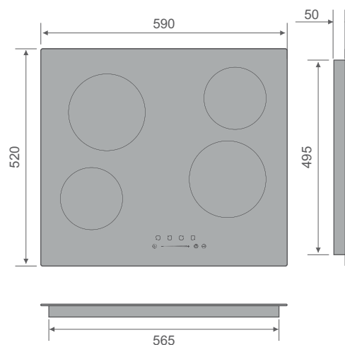
DRACO C604 SBK VIRGO C604 SBK ЭЛЕКТРИЧЕСКИЕ ВАРОЧНЫЕ ПАНЕЛИ
