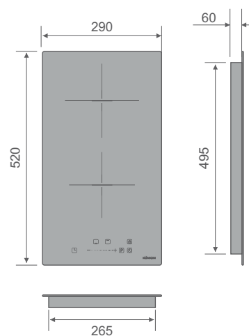
LACERTA I302 SBK ИНДУКЦИОННЫЕ ВАРОЧНЫЕ ПАНЕЛИ
