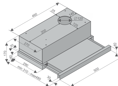
HELENA 50 / HELENA GLASS 50 ВСТРАИВАЕМЫЕ ТЕЛЕСКОПИЧЕСКИЕ
