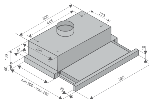
PIXEL ВСТРАИВАЕМЫЕ ТЕЛЕСКОПИЧЕСКИЕ
