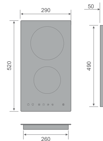
DRACO C302 TBK VIRGO C302 TBK ЭЛЕКТРИЧЕСКИЕ ВАРОЧНЫЕ ПАНЕЛИ
