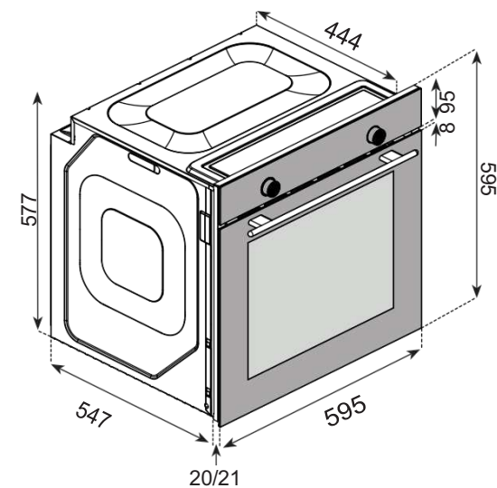
BARBERRY MR7/E9/E10 ДУХОВЫЕ ШКАФЫ
