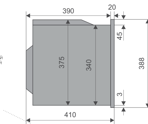
GTMB925BFG / GTMB925WG CB4
