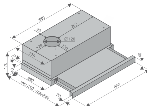
HELENA 60 / HELENA GLASS 60 ВСТРАИВАЕМЫЕ ТЕЛЕСКОПИЧЕСКИЕ
