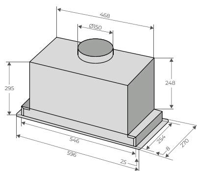
ALTEZZA ПОЛНОСТЬЮ ВСТРАИВАЕМЫЕ
