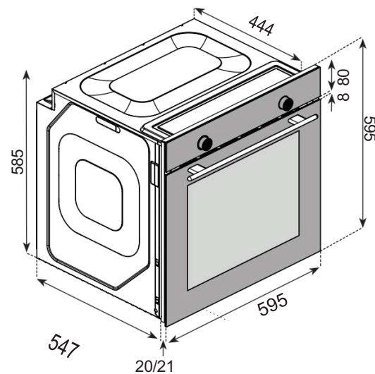
BARBERRY L10/LS10 ДУХОВЫЕ ШКАФЫ
