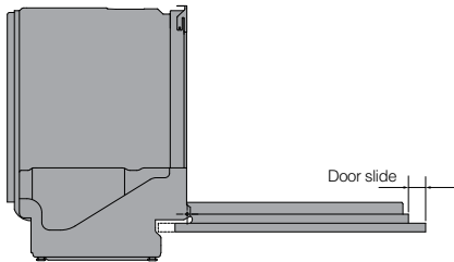
Монтаж со сдвижной дверцей (XL/XXL)
