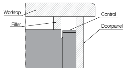
Нестандартный монтаж (ручка Gola)
