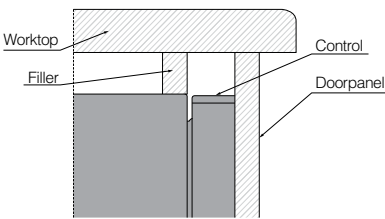
Нестандартный монтаж (ручка Gola)
