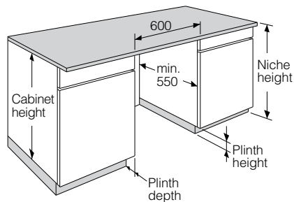
Размеры ниши
